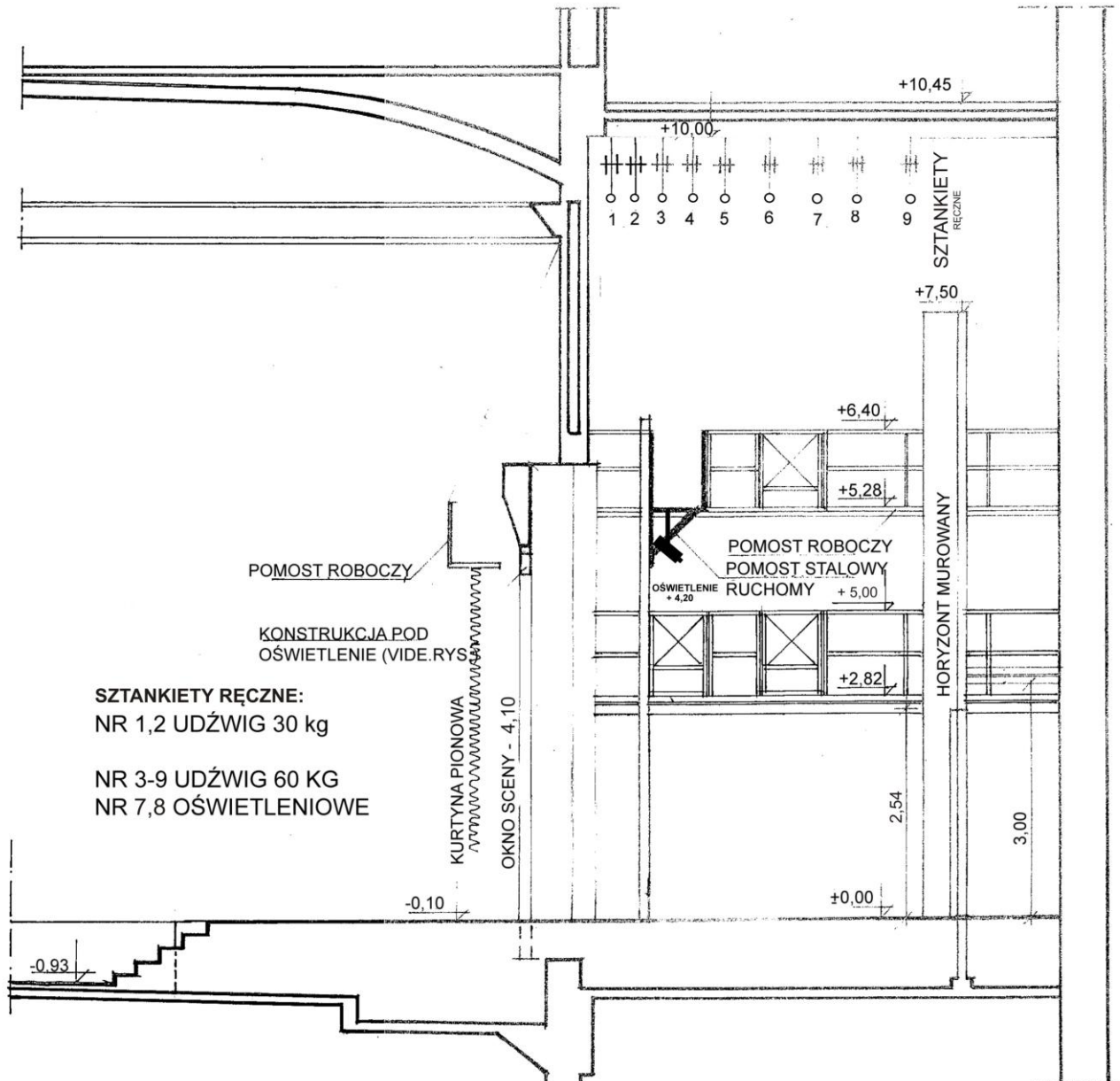
PRZEKRÓJ SALI TEATRALNEJ – RZUT NA KIESZEŃ SCENY
